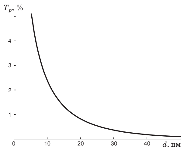
Рис. 1. Зависимость коэффициента пропускания T_p слоя золота на полиэтиленовой подложке от его толщины, рассчитанная для p -поляризованного излучения с \lambda = 130 мкм при угле падения 38^\circ 40' .
