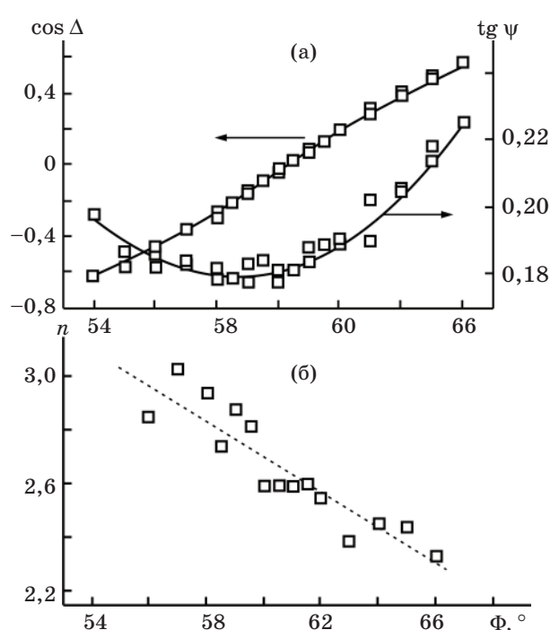
Рис. 3. Измеренные на длине волны 405 нм значения эллипсометрических параметров \cos \Delta и \text{tg } \psi (а) для образца 14 (квадратики) в сравнении с вычислениями в двухслойной модели пленки (сплошные кривые), а также показатель преломления n пленки, вычисленный в однослойной модели (б). Параметры двухслойной системы представлены в табл. 1.
