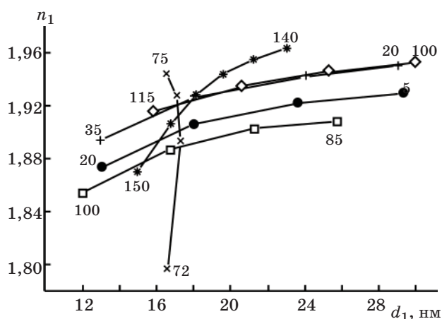
Рис. 4. Толщинные кривые для различных образцов (числа у кривых) на длине волны 579 нм. Цифры у засечек на кривых соответствуют толщине внутреннего слоя в нм.
