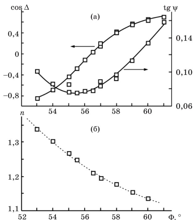
Рис. 2. Измеренные на длине волны 579 нм значения эллипсометрических параметров \cos \Delta и \text{tg } \psi (а) для образца 14 (квадратики) в сравнении с вычислениями в двухслойной модели пленки (сплошные кривые), а также показатель преломления n пленки, вычисленный в однослойной модели (б). Параметры двухслойной системы приведены в табл. 1.
